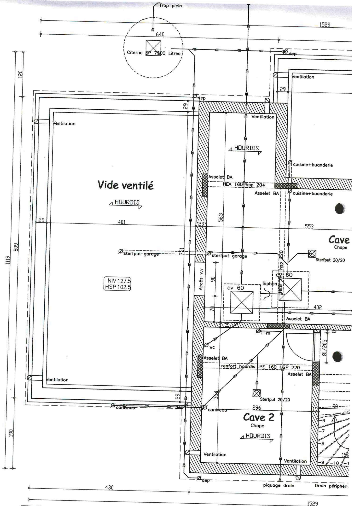
Plan Sous-Sol
